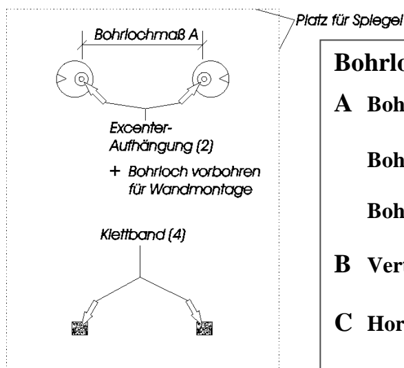
Abb.: 3 Wandansicht
